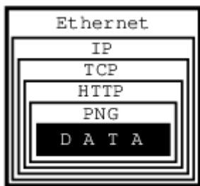
Рисунок 1. Уровни протоколов
