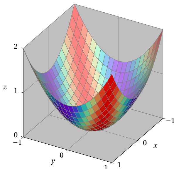
FIGURE 22 : La fonction ld.read_table3d()
