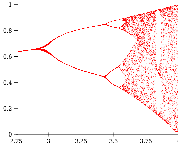
FIGURE 35 : Diagramme de bifurcation de la suite u_{n+1} = r u_n(1 - u_n)
