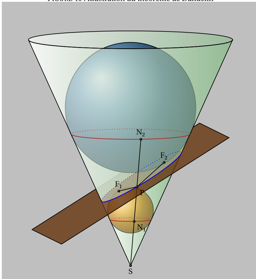
FIGURE 40 : Illustration du théorème de Dandelin
