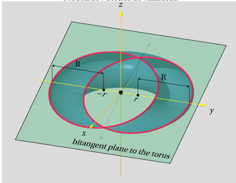
FIGURE 23 : Cercles de Villarceau
