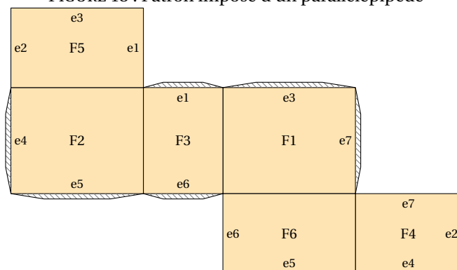
FIGURE 13 : Patron imposé d'un parallélépipède
