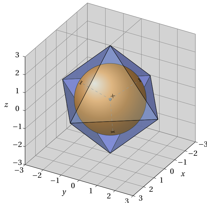
FIGURE 25 : Sphère inscrite dans un octaèdre avec projection du centre sur les faces
