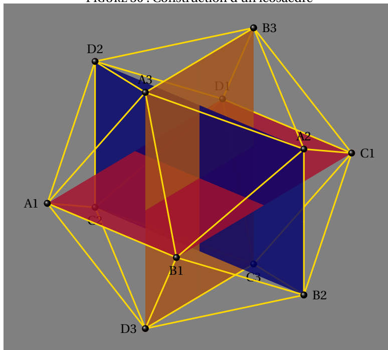
FIGURE 30 : Construction d'un icosaèdre
