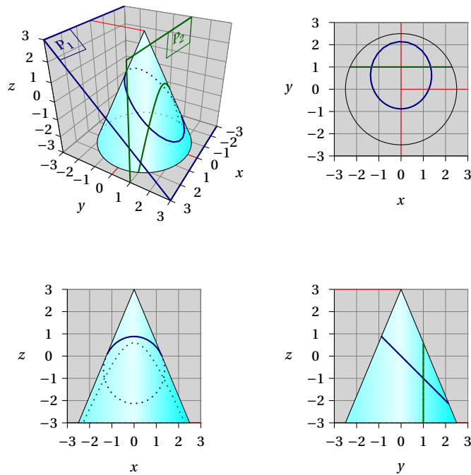
FIGURE 15 : Section de cône avec plusieurs vues
