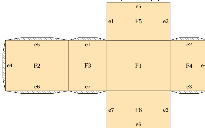
FIGURE 12 : Patron d'un parallélépipède
