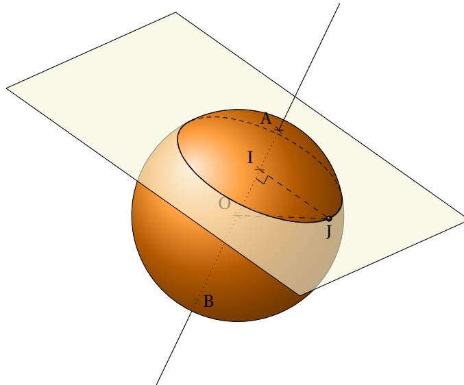
FIGURE 33 : Section de sphère sans Dscene3d()
