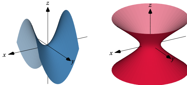
FIGURE 18 : Surfaces utilisant l'option addwall
