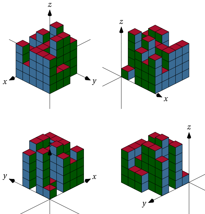
FIGURE 39 : Empilement de cubes
