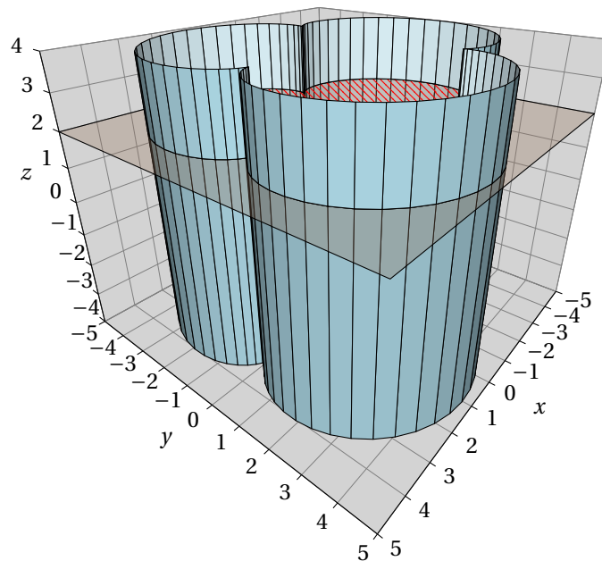
FIGURE 20 : Section d'un cylindre non circulaire
