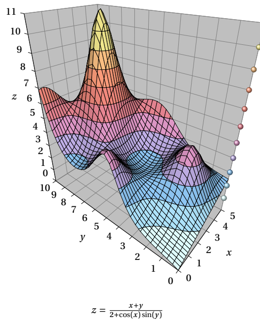
FIGURE 17 : Exemple de courbes de niveaux sur une surface
