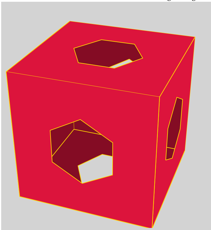
FIGURE 35 : Faces d'un cube trouées avec un hexagone régulier
