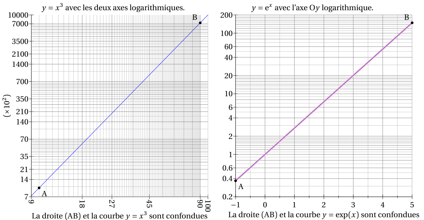
FIGURE 26 : Les deux autres cas de figure.
