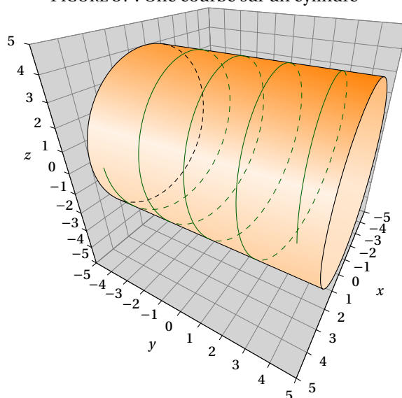
FIGURE 37 : Une courbe sur un cylindre
