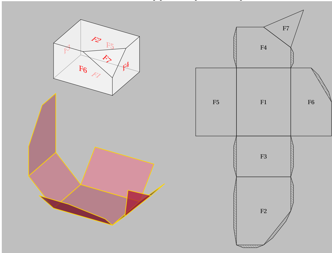
FIGURE 14 : Parallélépipède tronqué à demi déplié
