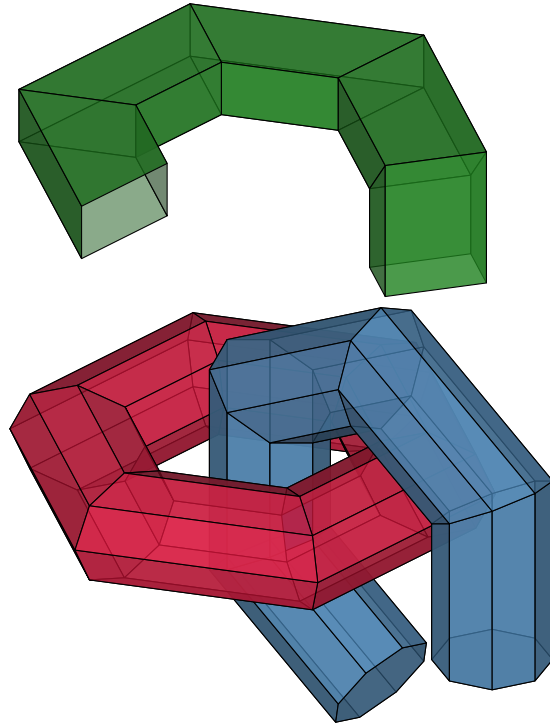
FIGURE 21 : Exemple avec line2tube et section2tube
