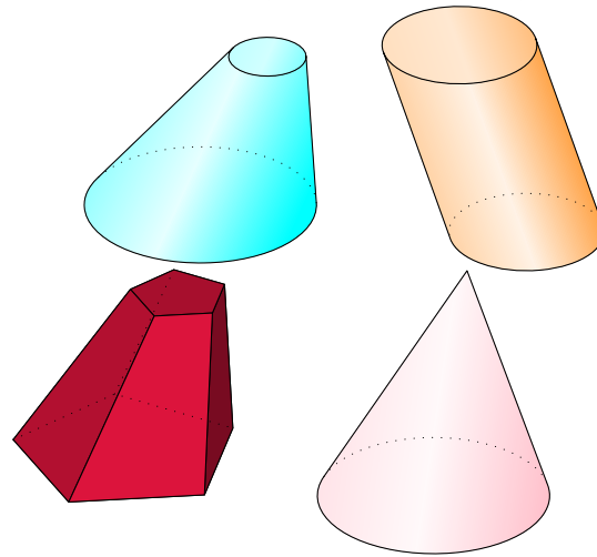
FIGURE 13 : Cône tronqué, pyramide tronquée, cylindre oblique
