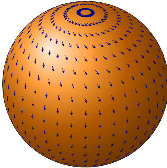
FIGURE 17 : Sur une sphère
