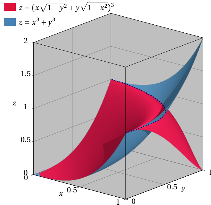
FIGURE 22 : Intersection de deux surfaces implicites
