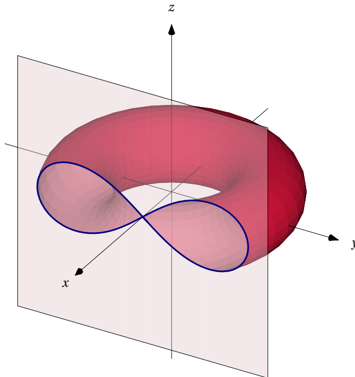
FIGURE 32 : Tore et lemniscate
