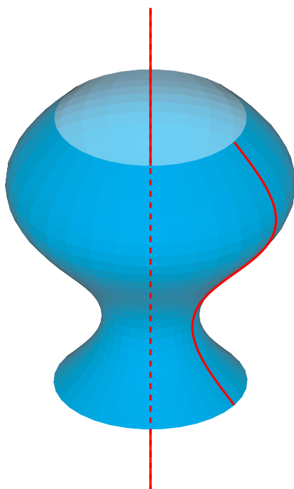
FIGURE 23 : Exemple avec rotcurve
