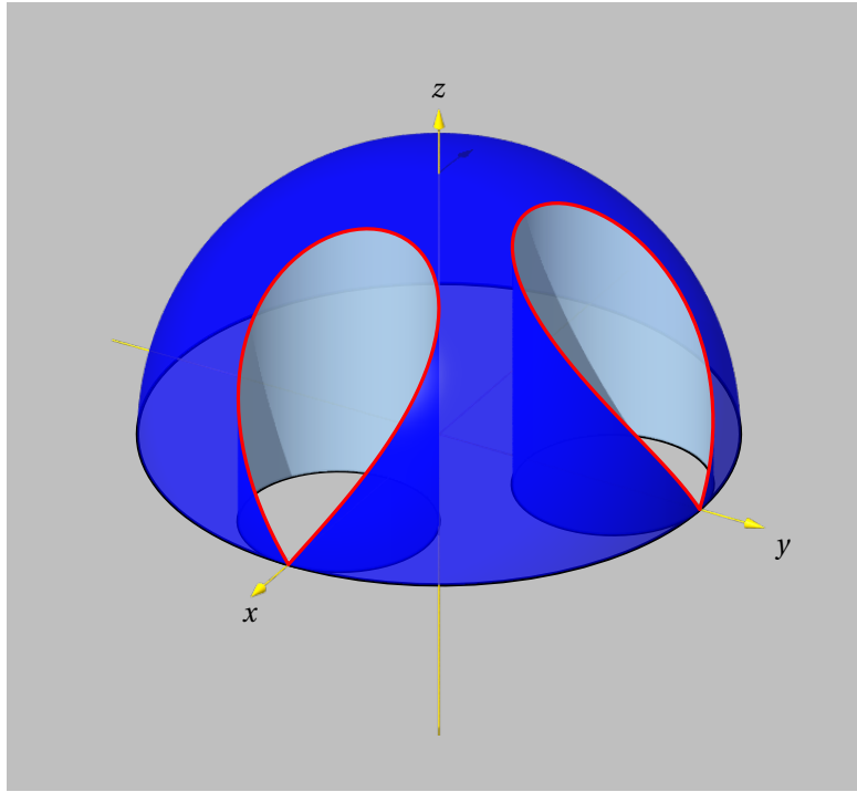
FIGURE 24 : Trous dans une demi-sphère
