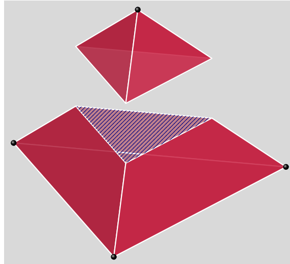
FIGURE 11 : Section d'un tétraèdre par un plan
