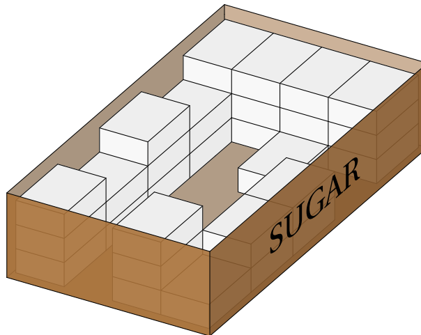
FIGURE 38 : Boite de morceaux de sucre
