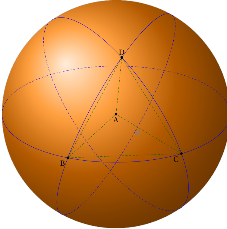
FIGURE 36 : Un tétraèdre avec la longueur des arêtes fixée
