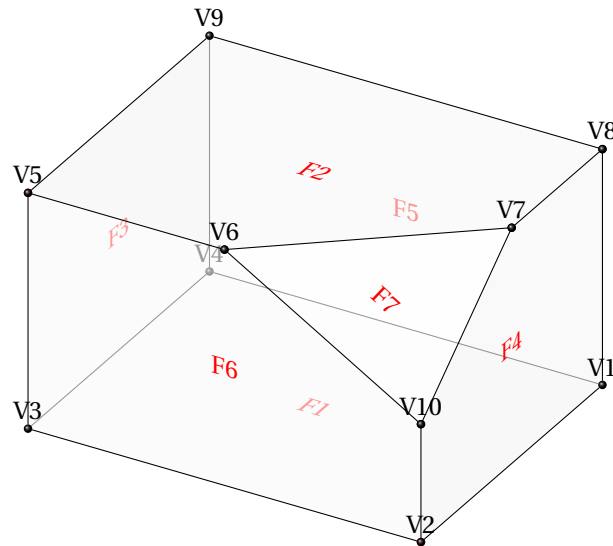
FIGURE 12 : Visualiser les faces et sommets d'un polyèdre
