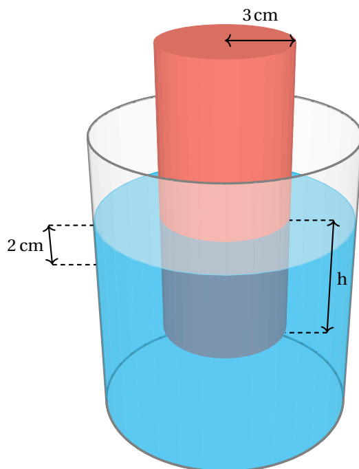
FIGURE 29 : Cylindre plein plongé dans de l'eau
