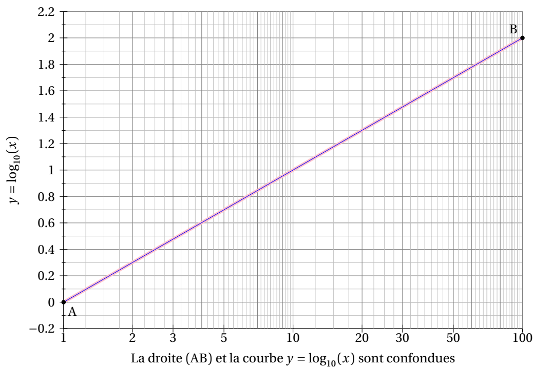
FIGURE 25 : Axe des x logarithmique
