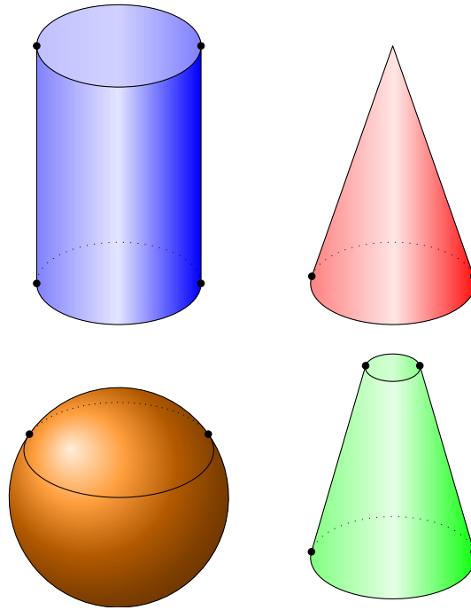
FIGURE 10 : Points de tangence
